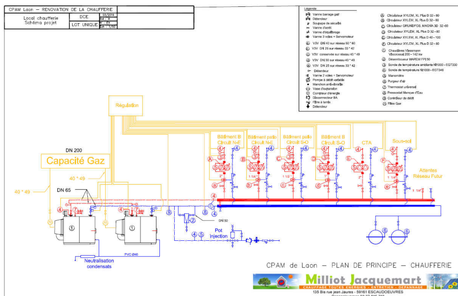
Schéma de chaufferie
